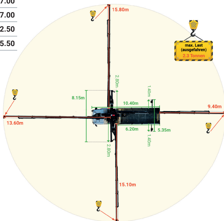
4-Achs Kranwagen: Belastung und Abstüzung
